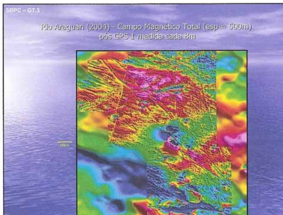
Fig. 57 – Superposição parcial de mapa aerogeofísico moderno de detalhe sobre o mapa da legenda anterior
