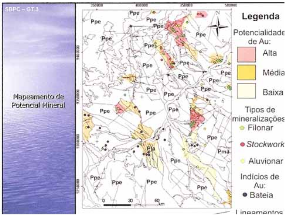
Fig. 67 – Exemplo de mapa potencial mineral obtido com apoio aerogeofísico e de imagens orbitais.
