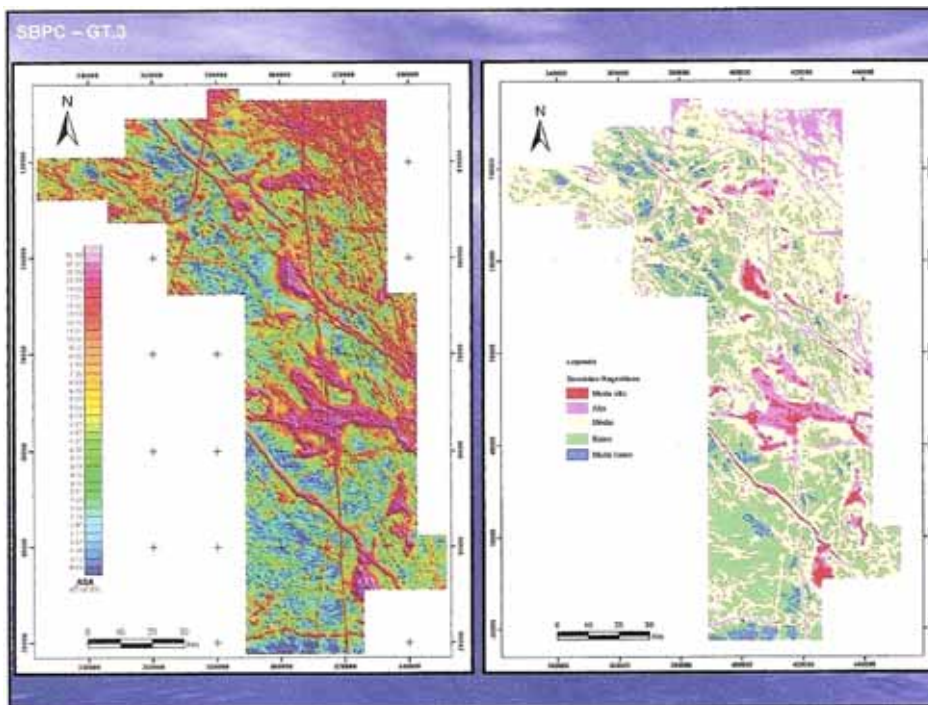
Fig. 58 – Mapa aeromagnético (esquerda) com respectiva interpretação geológica (direita)
