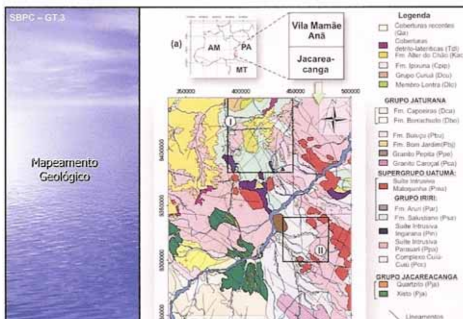
Fig. 66 – Exemplo de mapa geológico obtido com apoio da aerogeofísica e dos sensores remotos
