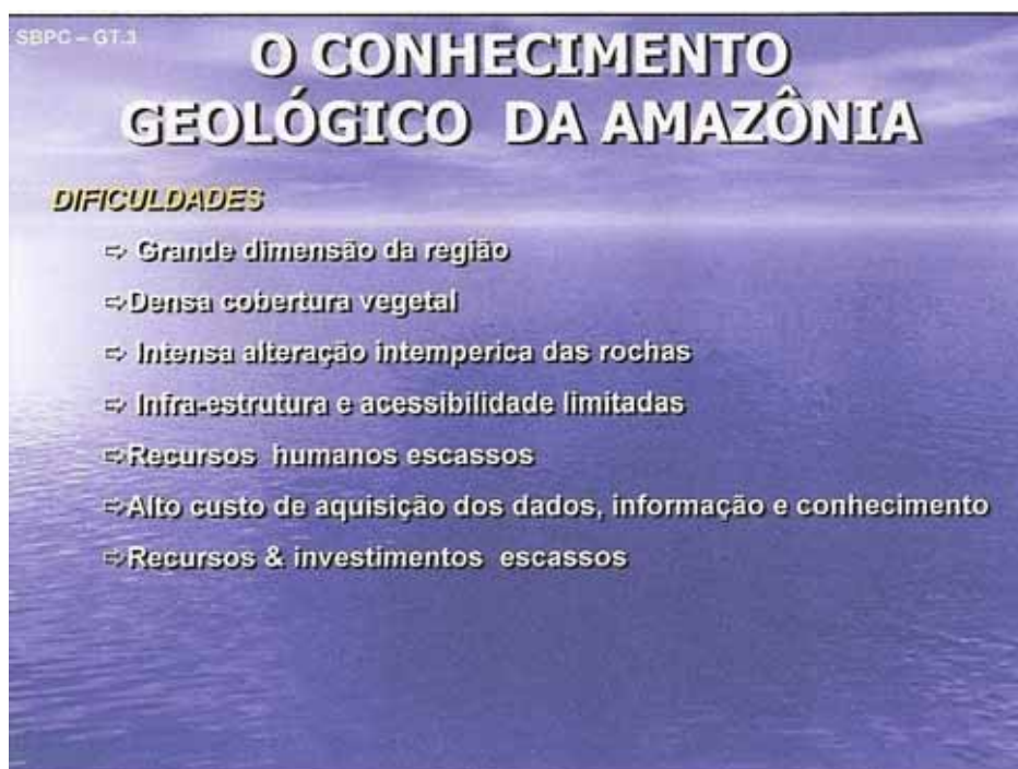
Fig. 05 – Dificuldade para o conhecimento geológico da Amazônia
