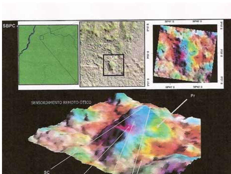
Fig. 65 – Mapa de relevo com definição de diferentes tipos de substâncias minerais obtido com auxílio de imagens hiperespectral do SIPAM
