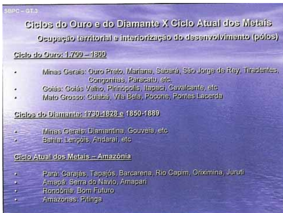
Fig. 14 – Ciclos do Ouro, Diamante e dos Metais
