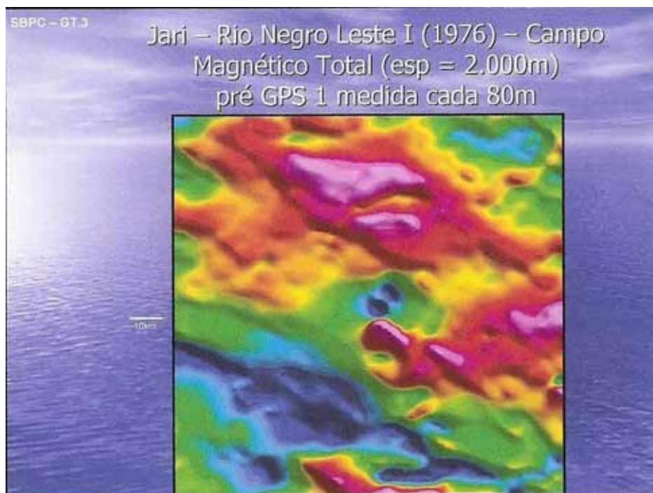
Fig. 56 – Mapa aeromagnético antigo (1976) sem detalhe e sem precisão.
